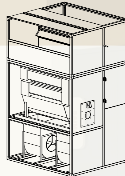
Gruppo Generatore - Power Unit
