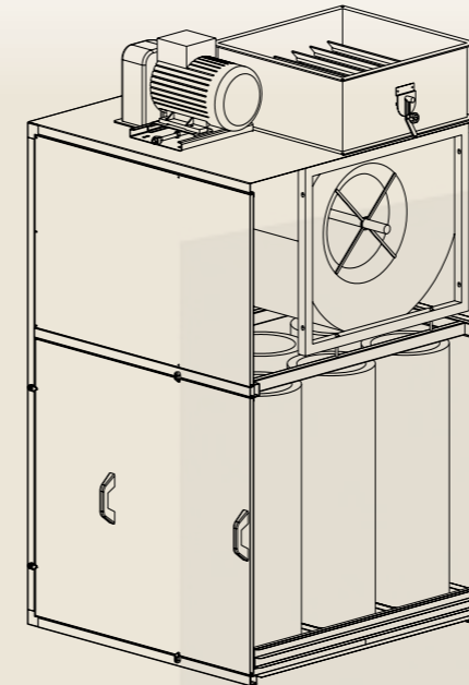
(optional) Depuratore ECA 12 a carboni attivi o versione SAIMA 12 con filtri a tasca. Activated cha-coal Exhaust Unit ECA 12 or SAIMA 12 type equipped with pocket filters.
